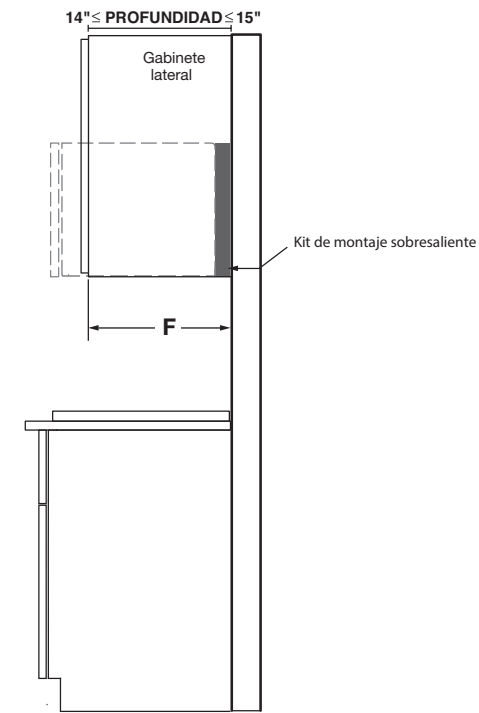
VISTA LATERAL
