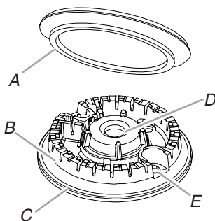
A. Chapeau de brûleur B. Orifices de brûleur C. Base du brûleur D. Ouverture du tube d'arrivée de gaz E. Tête de l'allumeur
