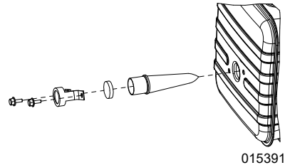
Figure 4-6. Tamis pare-étincelles
