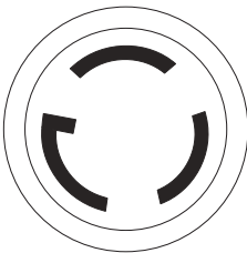
Figura 2-5. Receptáculo de 120 V CA, 30 A NEMA L5-30R
