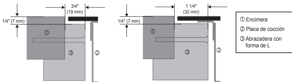
Abrazadera con forma de L (Delantera y trasera) Abrazadera con forma de L (Derecha e izquierda)
