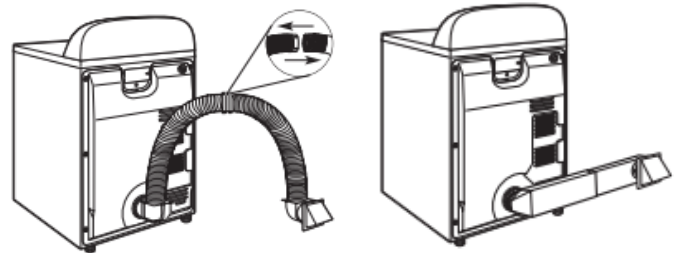
Installation au-dessus de la sècheuse Installation en péroscopie (également offerte avec un coude décalé)
