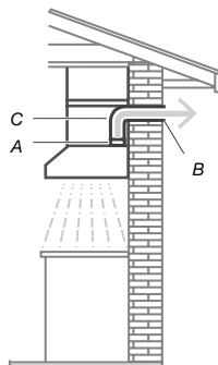
Descarga Horizontal
