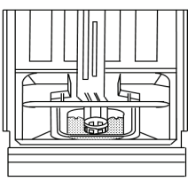
Filter Cup and Plate / Récipient et plaque du filtre de rinçage / Taza del filtro y la placa
