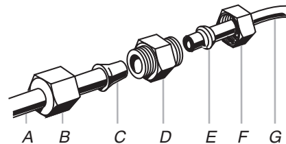
A. Tuyau d'eau dur réfrigérateur B. Écrou (fourni) C. Renflement D. Raccord (à acheter) E. Virole (à acheter) F. Écrou (à acheter) G. Canalisation du domicile
